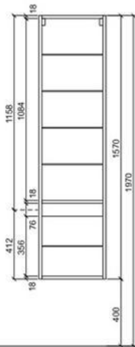
Nárys
