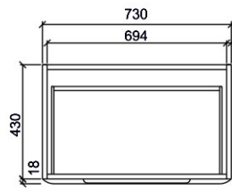
Půdorys
