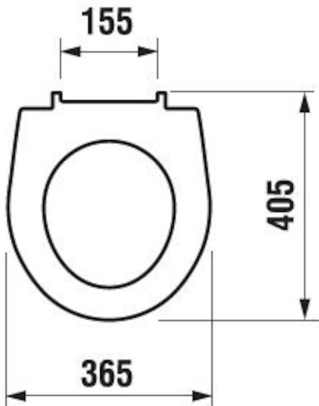
duroplastové sedátko pro kombiklozety
